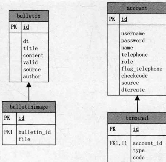
图 12.3 公告和用户 E-R 图
