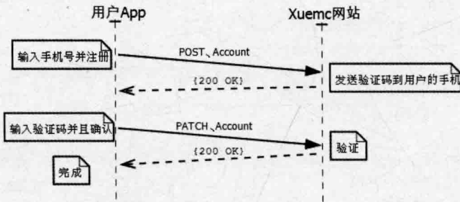
图 12.6 用户注册及验证流程
