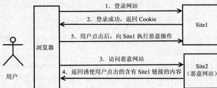
图 7.2 CSRF 的基本原理图
