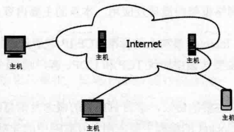
图 2.1 Internet 抽象图
