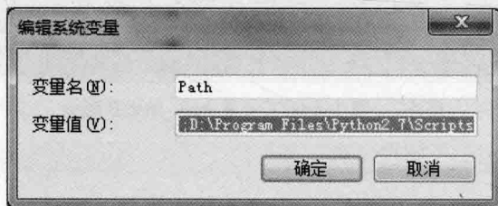
图 5.6 easy_install 安装
