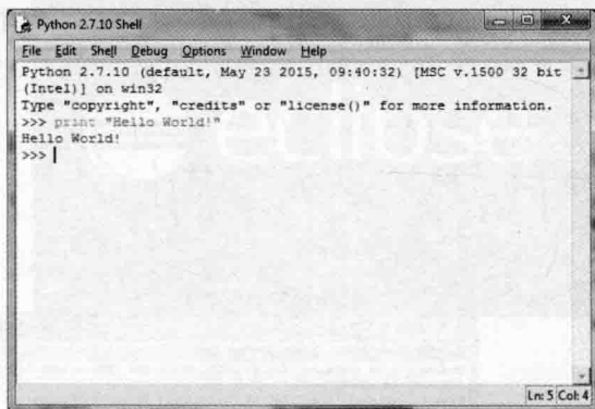
图 1.6 IDLE 界面
