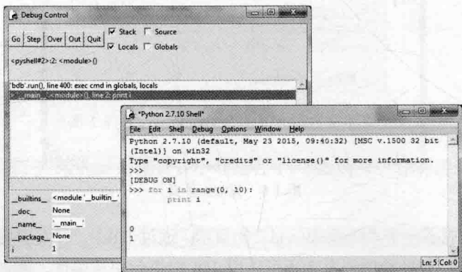
图 1.7 在 IDLE 中调试 Python 语句
