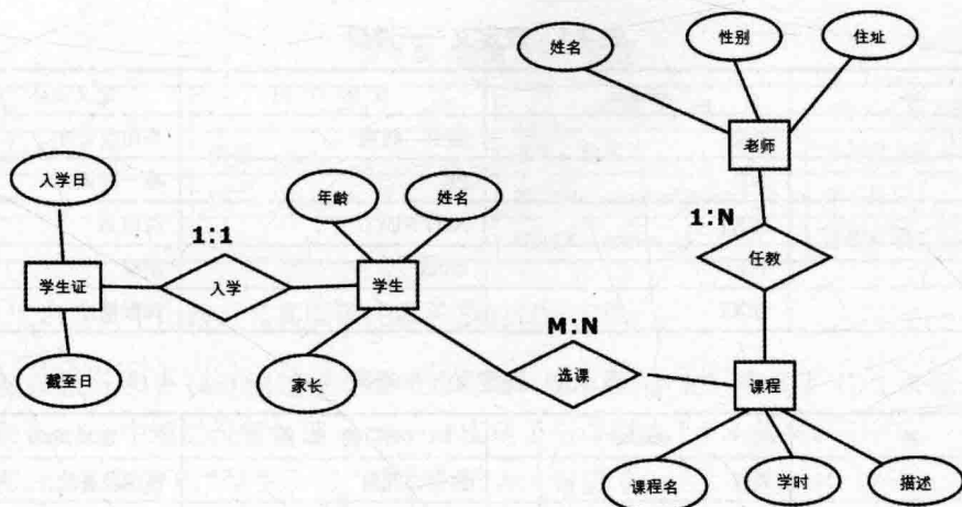
图 4.2 学校系统的 E-R 图示例
