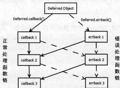
图 9.3 Defer 函数链的调用流程
