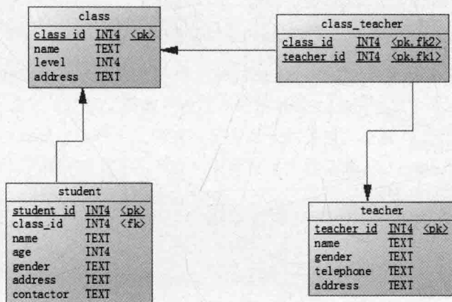
图 8.7 学校老师、班级、学生子系统的 E-R 图
