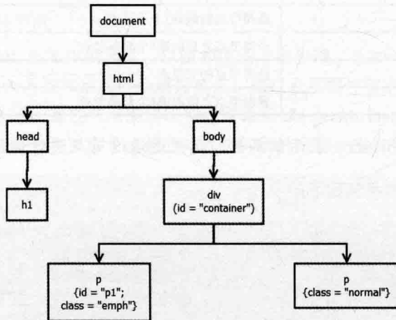
图 3.12 DOM 树示例
