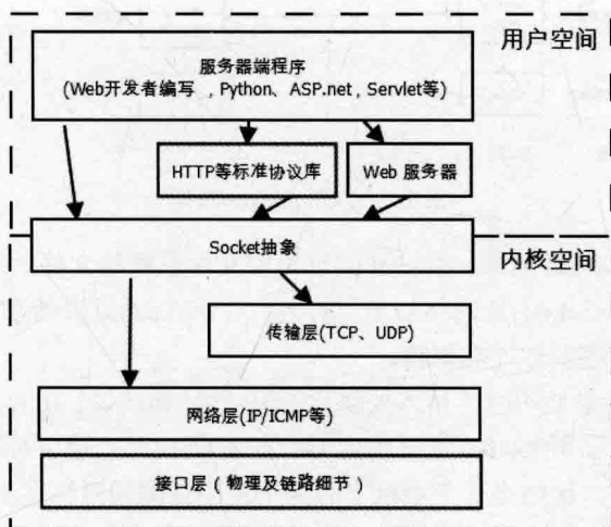
图 2.6 Socket 抽象
