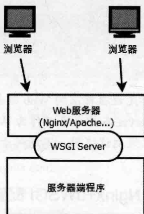
图 5.9 WSGI 的作用
