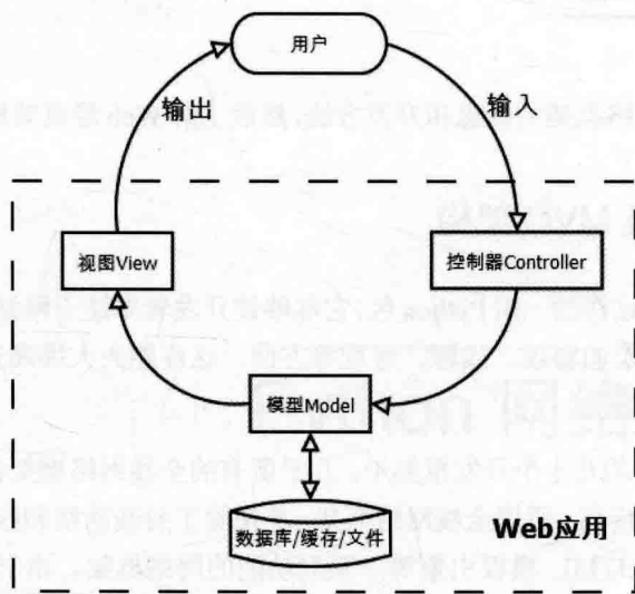
图 5.1 MVC 架构图
