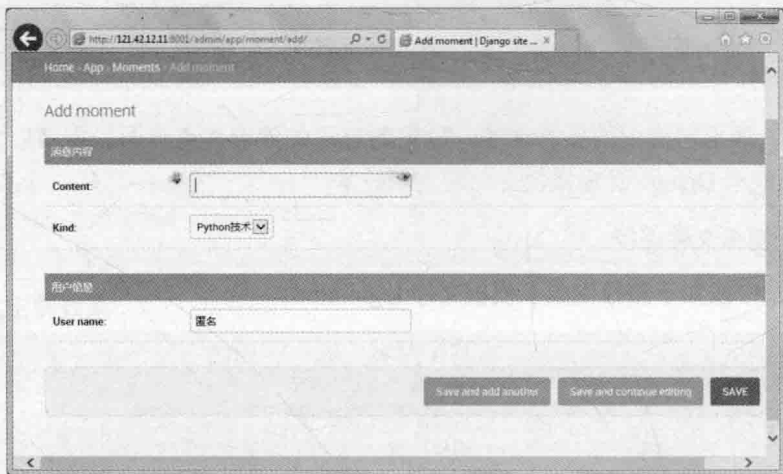
图 6.6 字段分组
