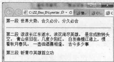
图 3.3 显示效果
