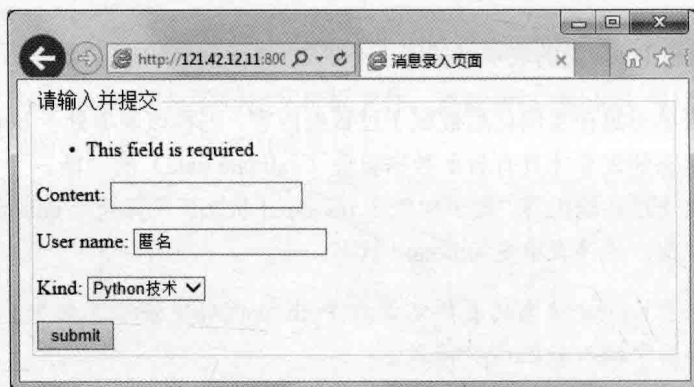
图 6.4 渲染结果
